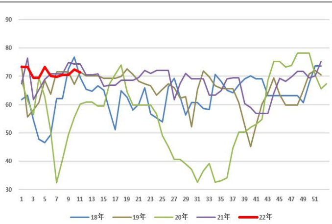
图 19：DMF 开工率
