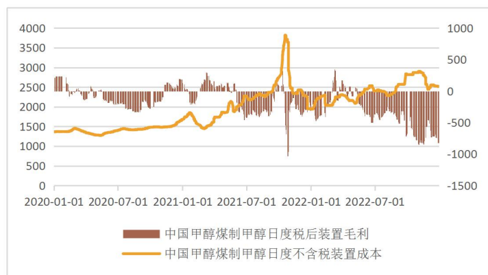
图 7：煤制甲醇现金流：元/吨
