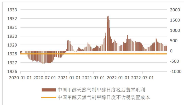
图 8：天然气制甲醇现金流：元/吨
